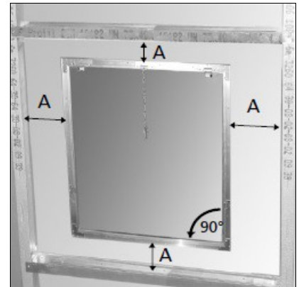
A = min. 8mm, max. 100mm
