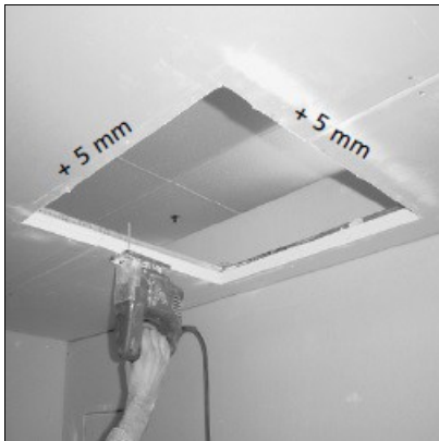
Cotes de montage + 5mm
